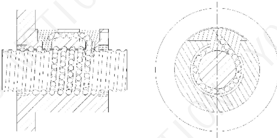
Fig 1.6.3 V-Type Nut
